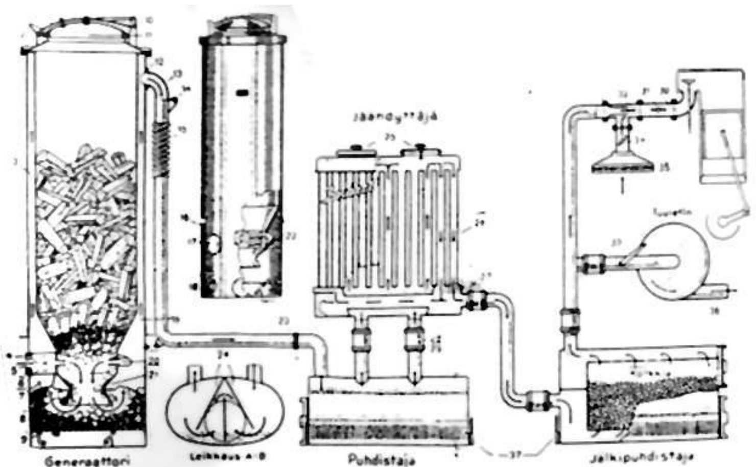
42 kuva. Imbert-puukaasutin. 1 Täyttölaukku, 2 Kannen sulkurengas, 3 Sisävaippa, 4 Laippa, 5 Ilma- ja sytytysaukko, 6 Ilmanjakokammio, 7 Luukku, 8 Puuhiliä, 9 Arina, 10 Salpa, 11 Kanssi, 12 Putkenlaippa, 13 Putkimutka, 14 Huuhtelutulppa, 15 Taipuvaa putkea, 16 Kannatinrauta, 17 Luukun kanssi, 18 Ravistusvarsi, 19 Kehittimen alakammio, 20 Suutin, 21 Tulipesä, 22 Tulistusputki, 23 Putkilaippa, 24 Väliseinämät, 25 Jäähdyttäjän kannet, 26 Jäähdytysputket, 27 Jäähdyttäjän alakammio, 28 Kumiliittimet, 29 Liitospuristimet, 30 Kaasuputki, 31 Kaasuläppä, 32 Sekoitusventtiili, 33 Imurin lippö, 34 Ilmaläppä, 35 Ilmanpuhdistaja, 36 Imurin poistoputki, 37 Vedenpoistohanat.
